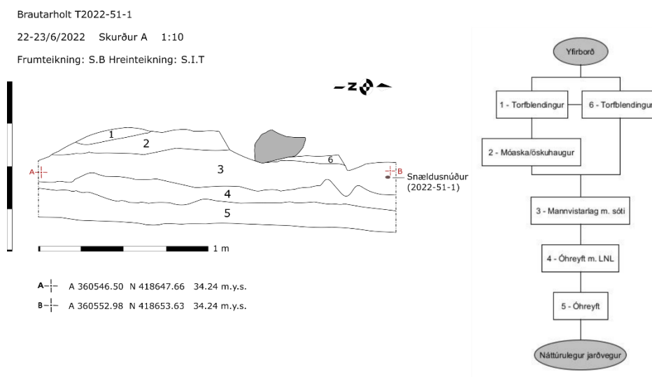
Mynd 10. Sniðteikning af vestursniði í skurði A, ásamt flæðiriti. Steininn á teikningunni er hluti af grjóthleðslunni sem eigandinn kom niður á, mannvirki [2]. Búið var að raska jarðlögum vinstra megin við grjótið.
